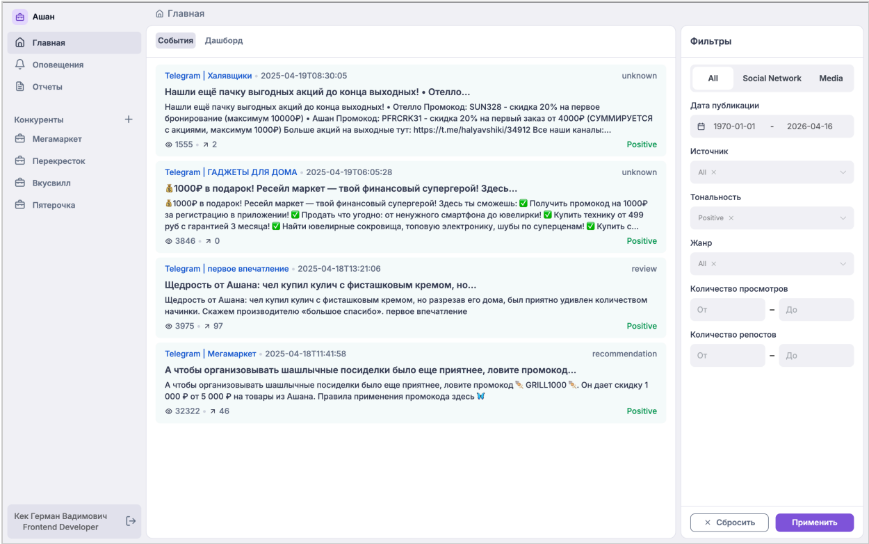
Рисунок 2 — Главная страница системы с текстовой навигацией и фильтрами
